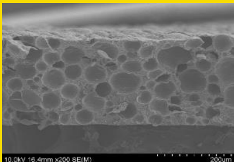
オプティマス塗布面の断面図 / 標準塗布膜厚 250µm
